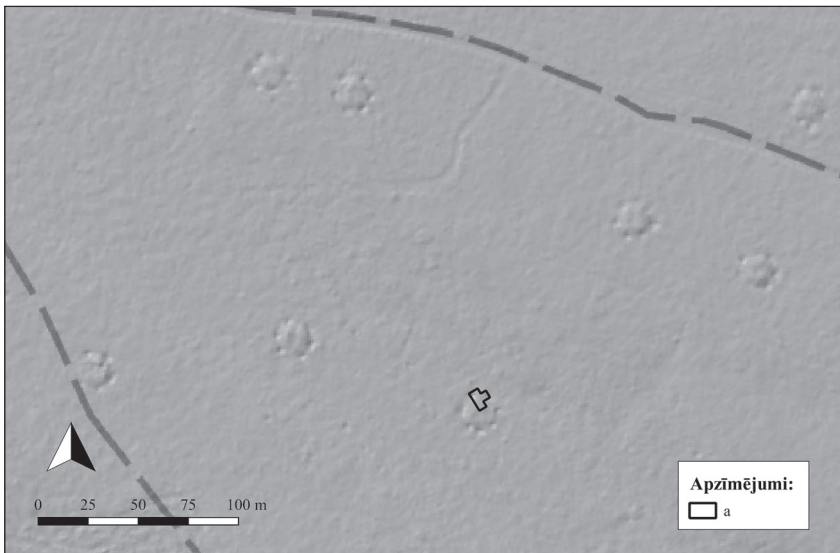
2. att. LiDAR datos redzami kokogļu ieguves uzkalniņi pie Apšuciema ar norādītu izrakumu vietu: a – izrakumu laukums (sagatavojusi E. Guščika; kartes pamatā: LIDAR HS. LIDAR DEM ēnojuma mozaīka ar 1 m izšķirtspēju, izgatavota no LĢIA LiDAR datiem. LU ĢZZF WMS; TOPO 10 LV. LĢIA LR topogrāfiskā karte mērogā 1:10 000. LU ĢZZF WMS; pieejami: http://www.geo.lu.lv/kartes , http://kartes.geo.lu.lv (skatīts 03.02.2019.))
